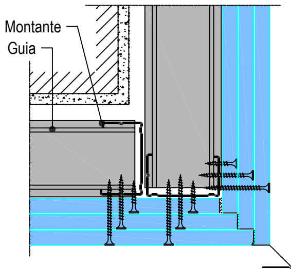
1 CANTO EXTERNO W628 SEM ESCALA
