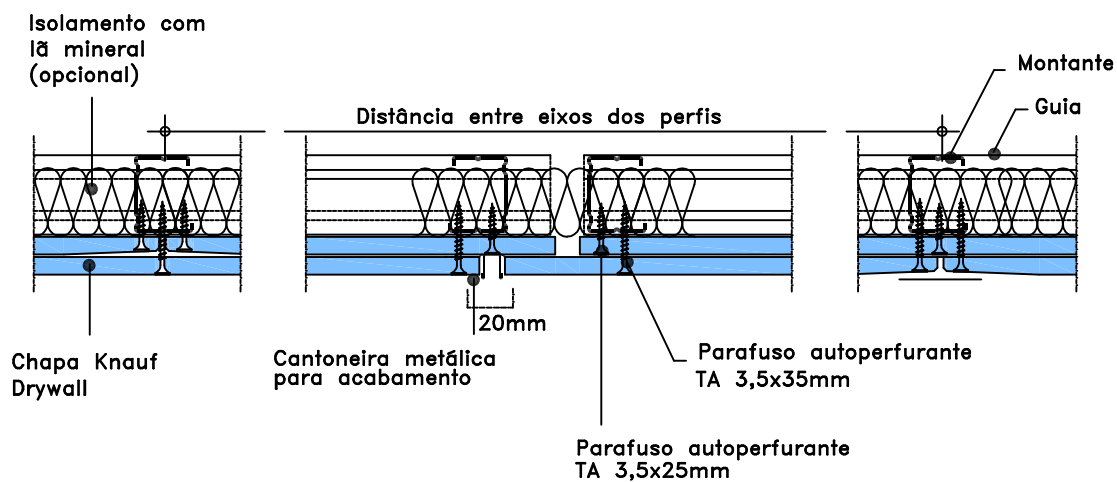
1 CORTE HORIZONTAL – JUNTA DE DILATAÇÃO EM W626 SEM ESCALA
