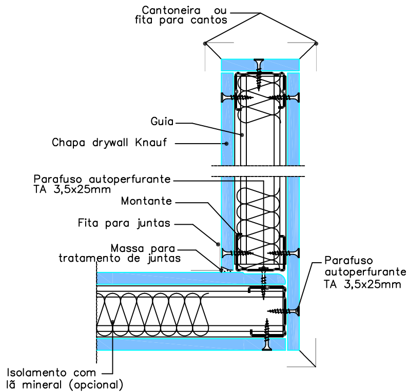
1 DETALHE – ENCONTRO DE PAREDE EM L – W111 SEM ESCALA
