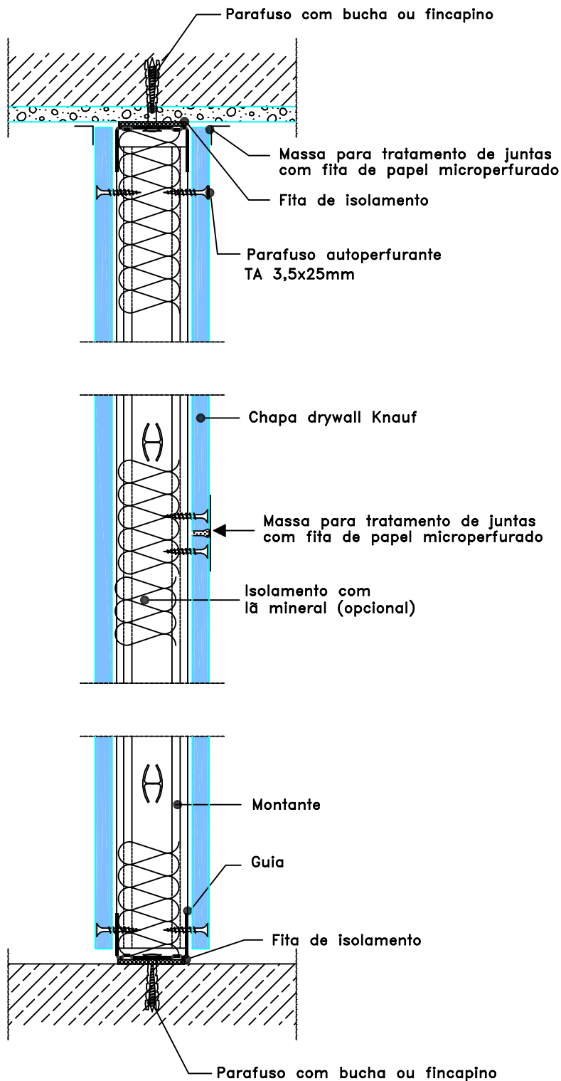
1 CORTE VERTICAL - W111 SEM ESCALA
