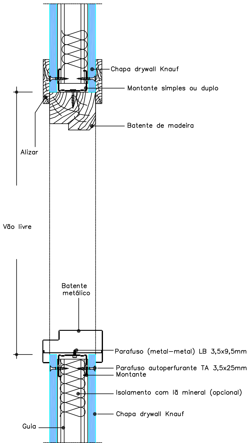
1 DETALHE – CONFIGURAÇÃO DE PORTA – W111 SEM ESCALA
