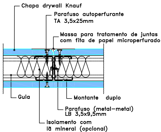
2 DETALHE – JUNTA DE CHAPAS ESTRUTURA DUPLA – W111 SEM ESCALA
