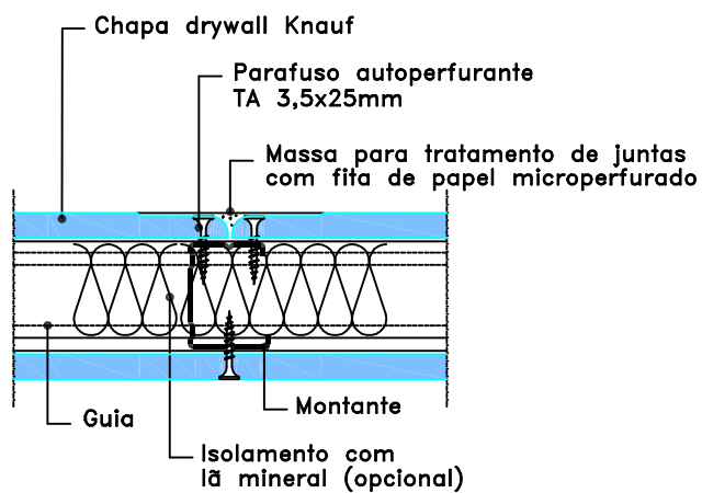
1 DETALHE – JUNTA DE CHAPAS ESTRUTURA SIMPLES – W111 SEM ESCALA
